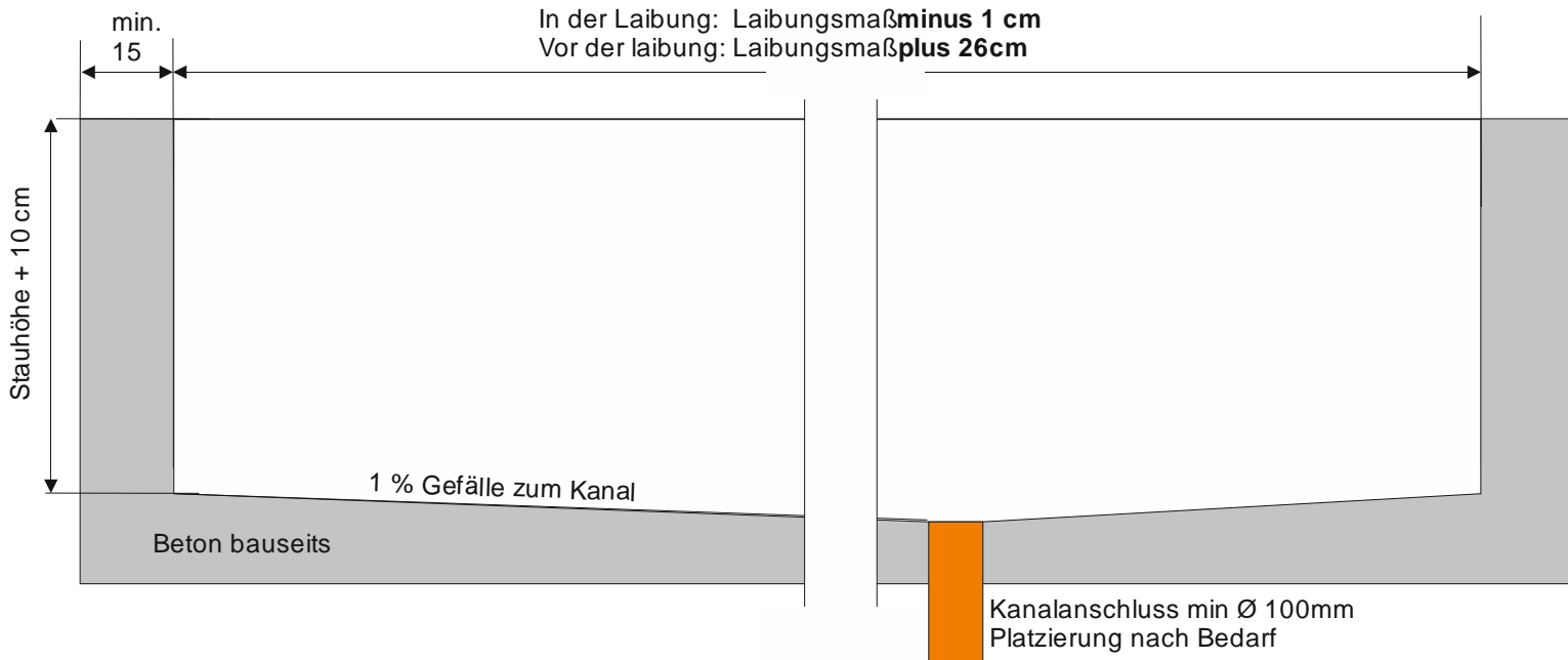
Schnitt A-A
